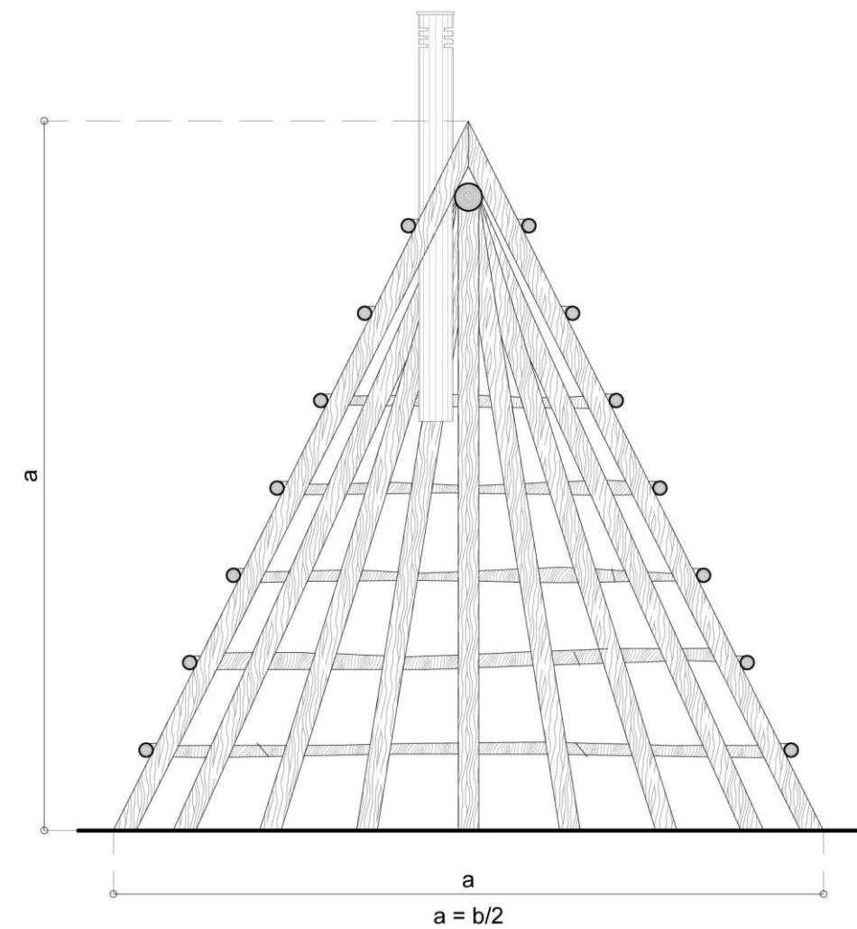
Figura 5 – Casone principale. Sezione trasversale A-A.
