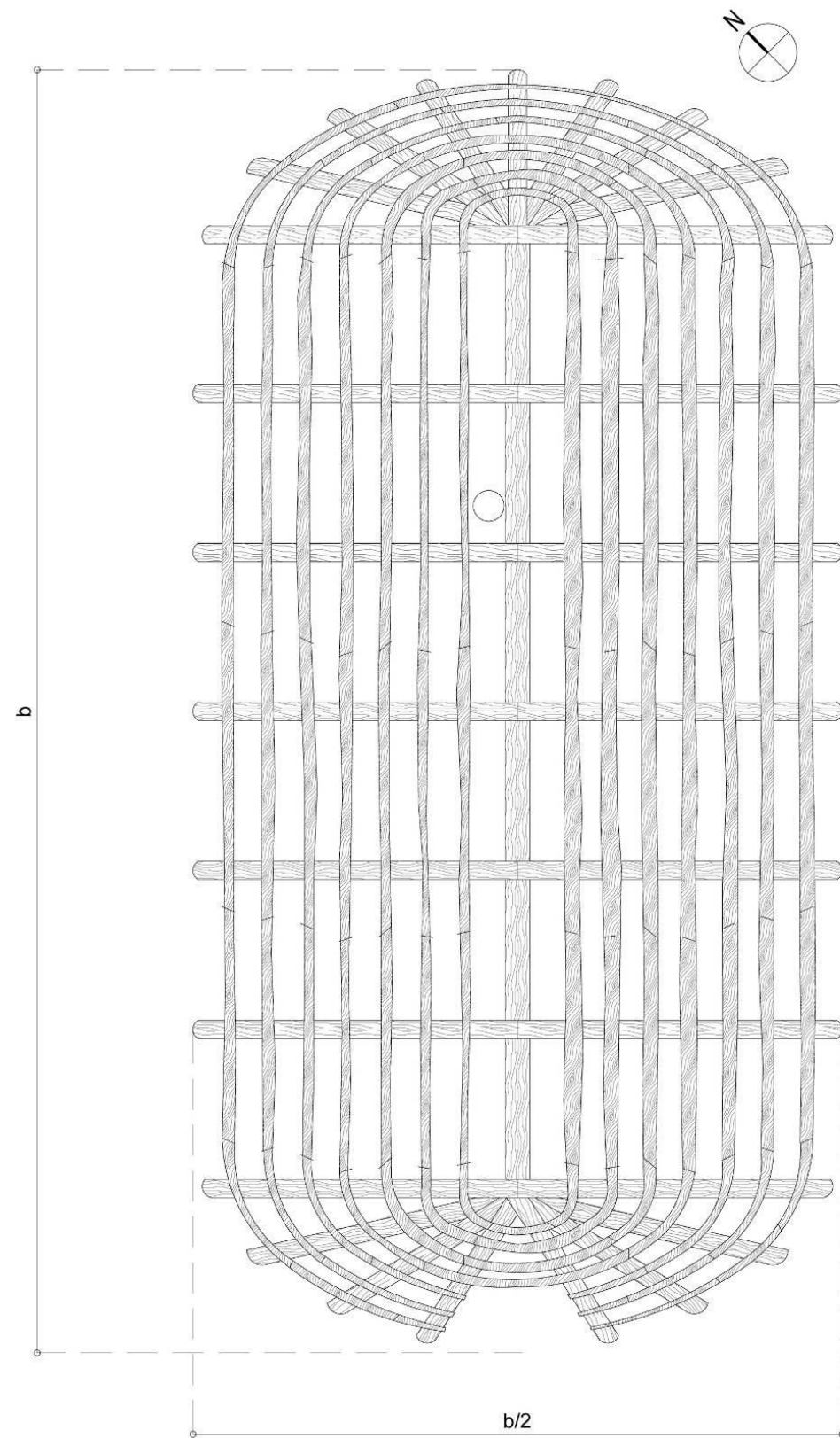
Figura 1 – Casone principale. Pianta orditura strutturale.
