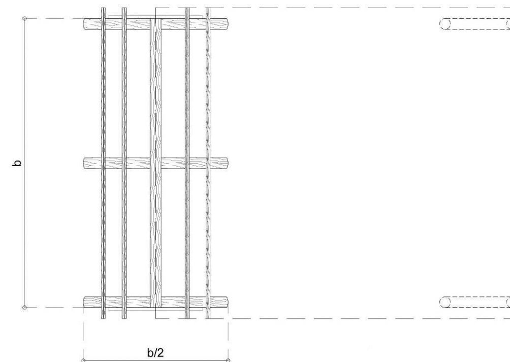
Figura 19 – Tesora. Pianta.
