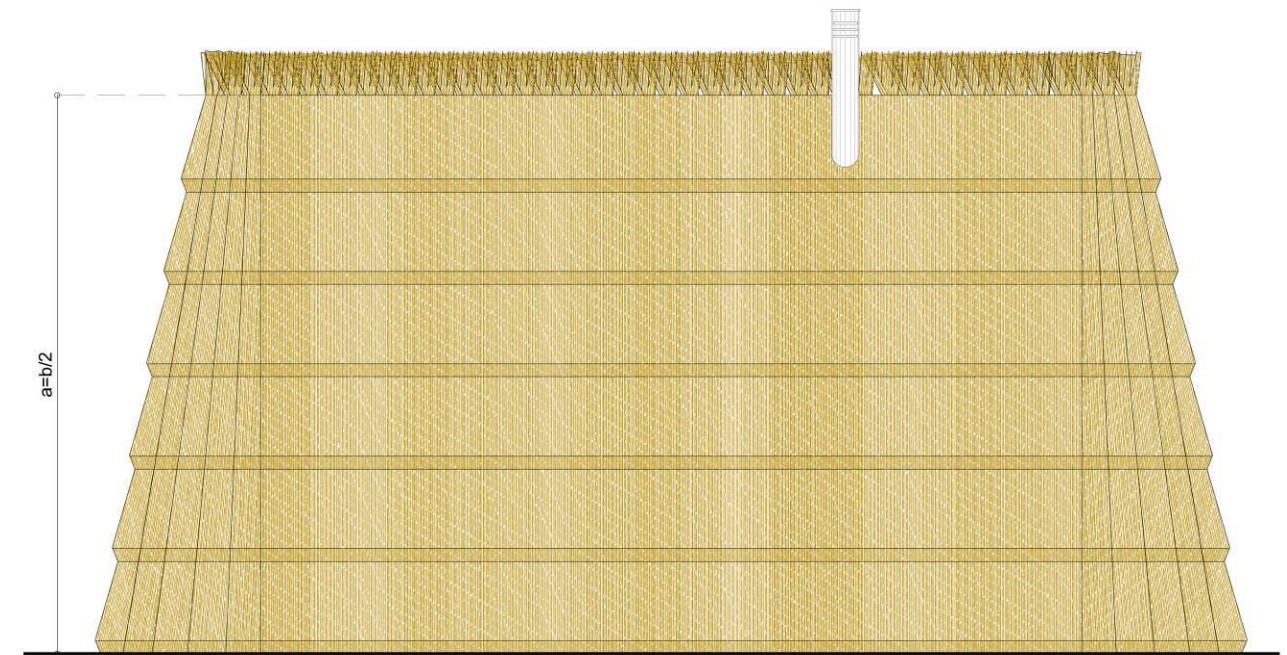
Figura 8 – Casone principale. Sezione longitudinale B-B.
