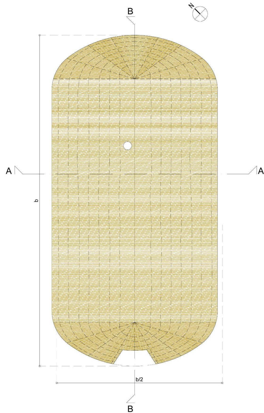
Figura 3 – Casone principale. Pianta copertura.
