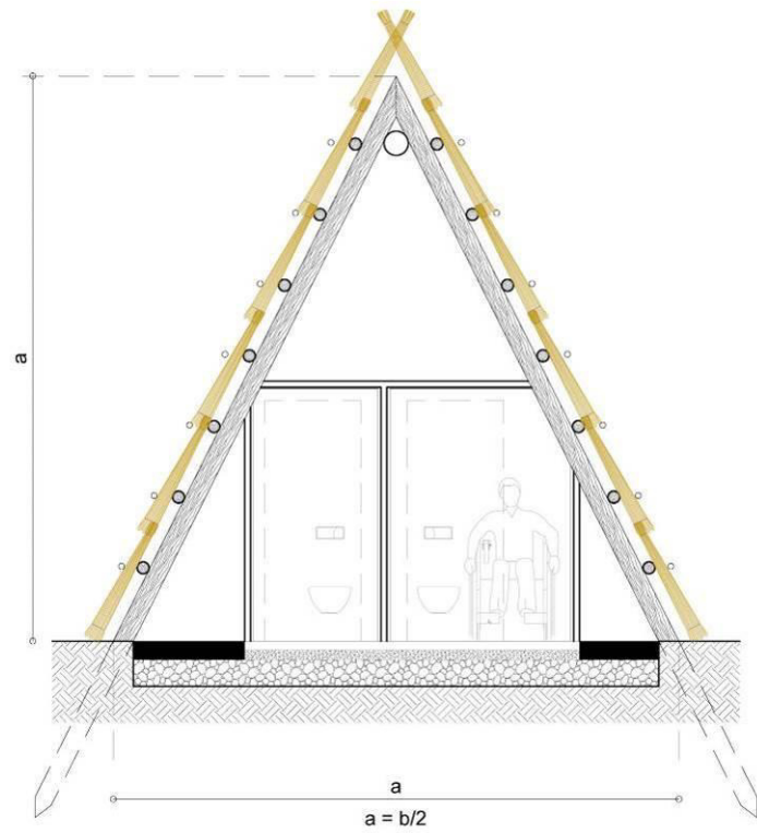
Figura 15 – Casone secondario. Sezione trasversale A-A.
