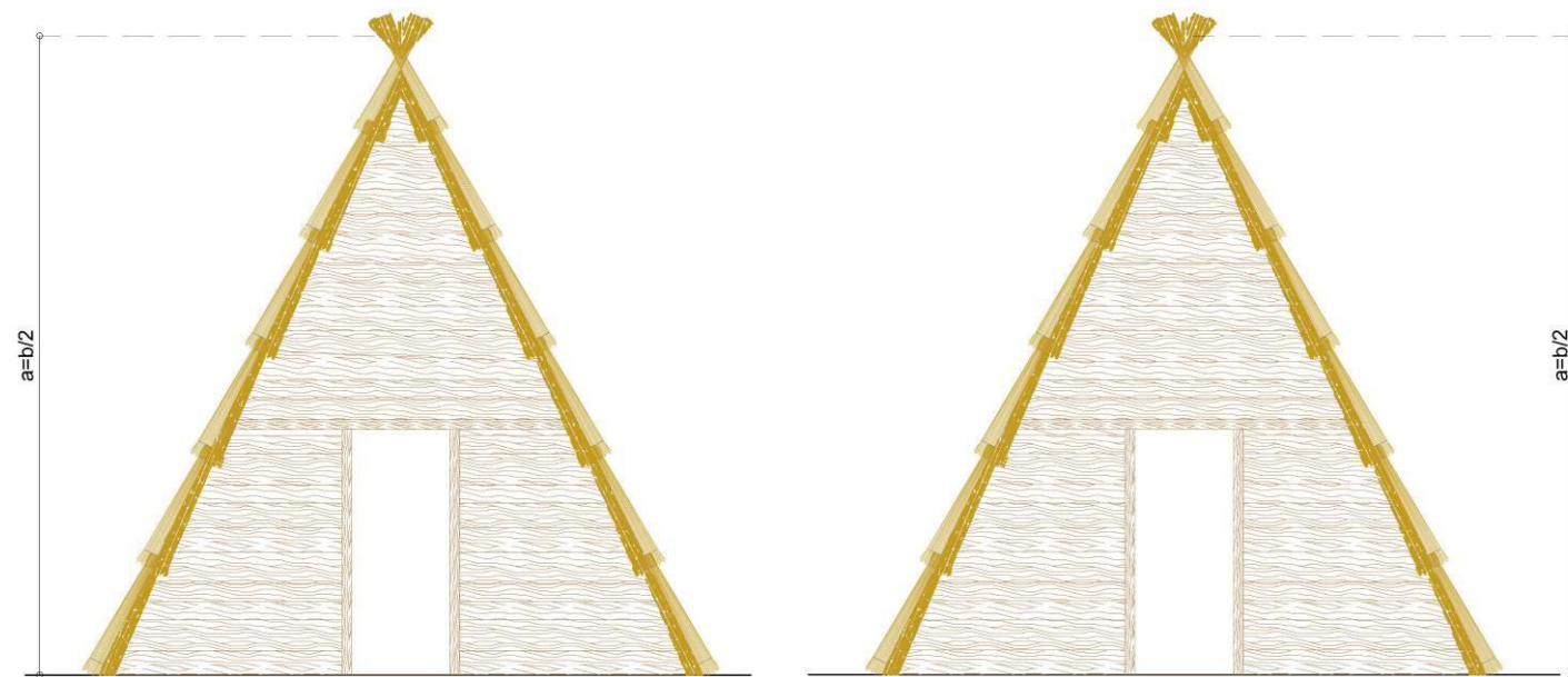
Figura 16 – Casone secondario. Prospetti dei lati corti o testate.
