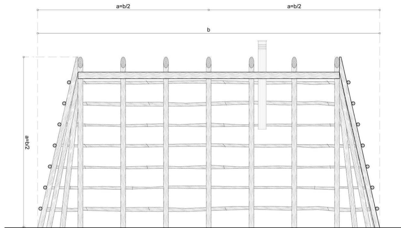
Figura 6 – Casone principale. Sezione longitudinale B-B.
