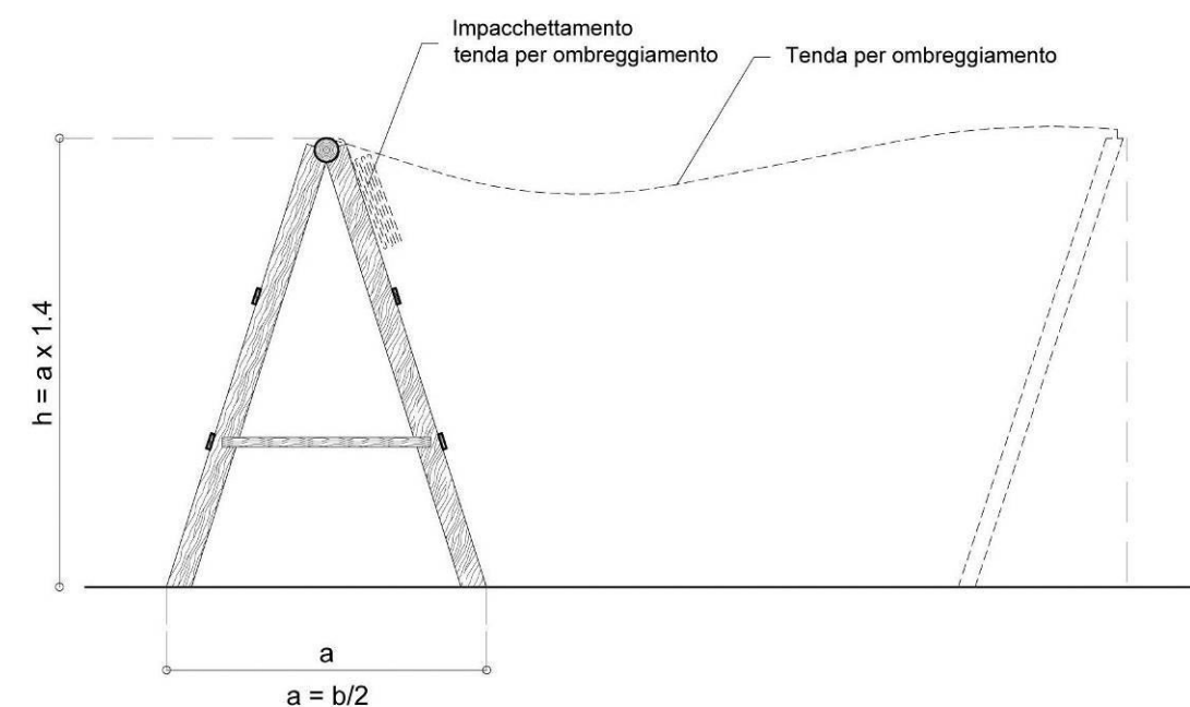
Figura 20 – Tesora. Sezione trasversale.
