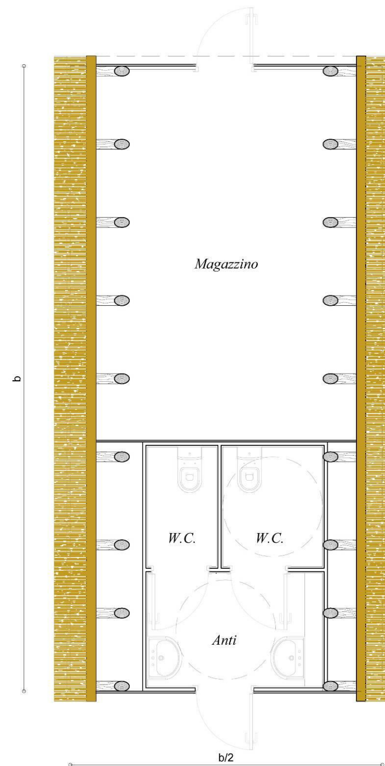
Figura 12 – Casone secondario. Pianta (suddivisione interna non prescrittiva).
