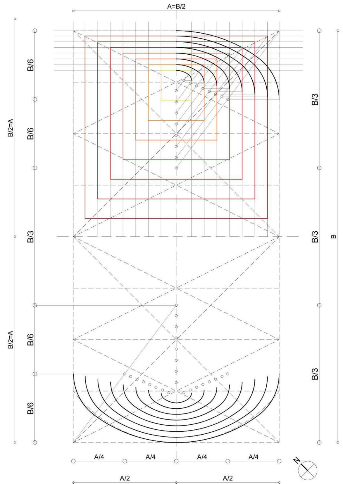
Figura 11 – Casone principale. Schema geometrico di coordinamento proporzionale.
