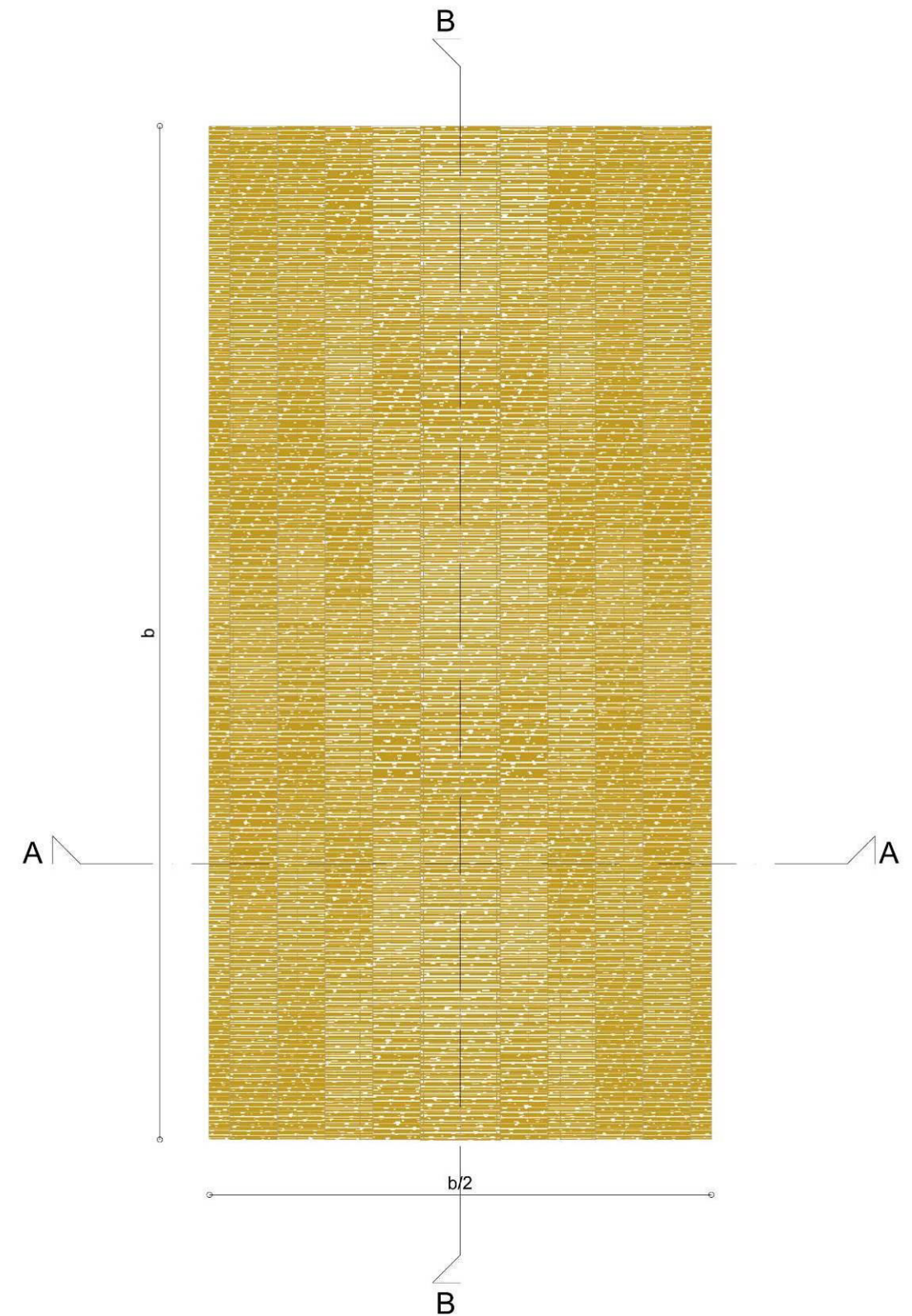
Figura 14 – Casone secondario. Pianta copertura.
