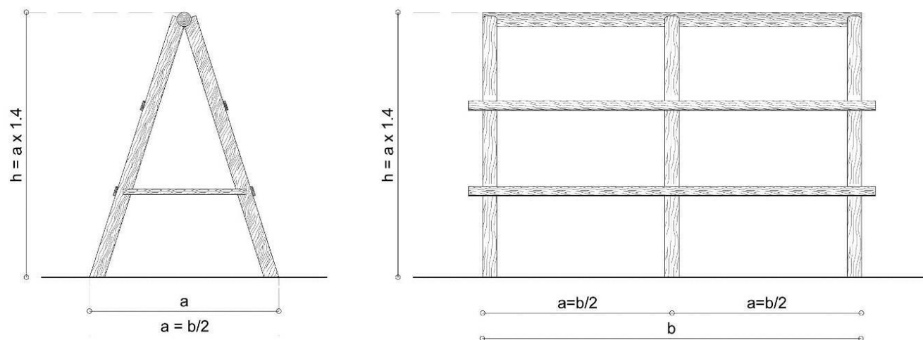
Figura 18 – Tesora. Prospetti frontale e laterale.
