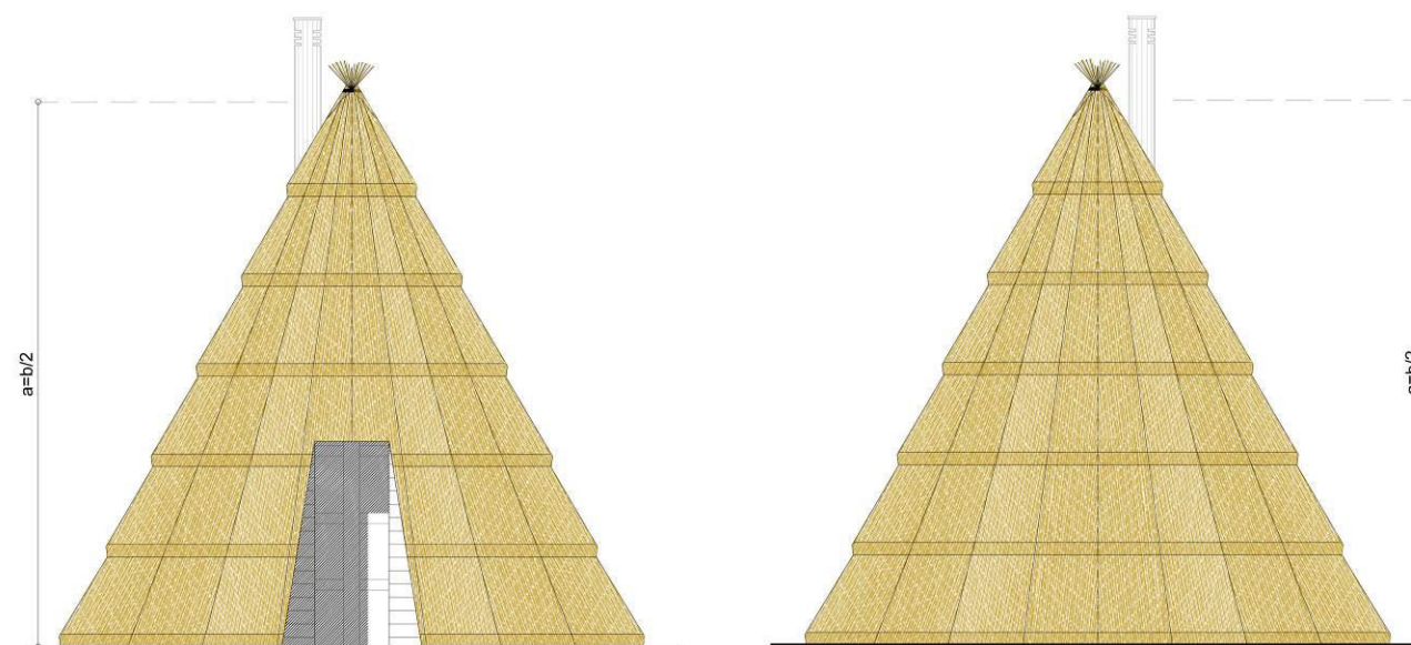
Figura 7 – Casone principale. Prospetto frontale e del retro.
