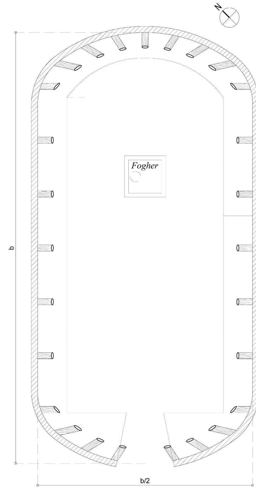
Figura 2 – Casone principale. Pianta.
